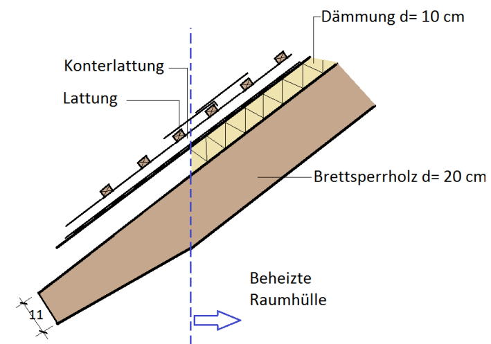
Variante ohne Dachüberstand
