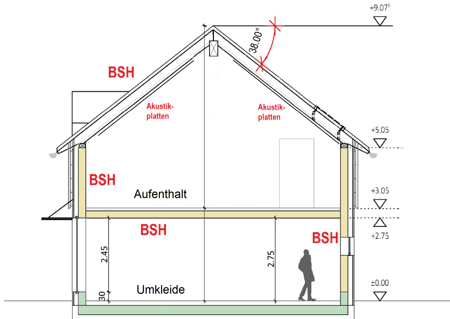
Schnitt Umkleide-Aufenthalt
