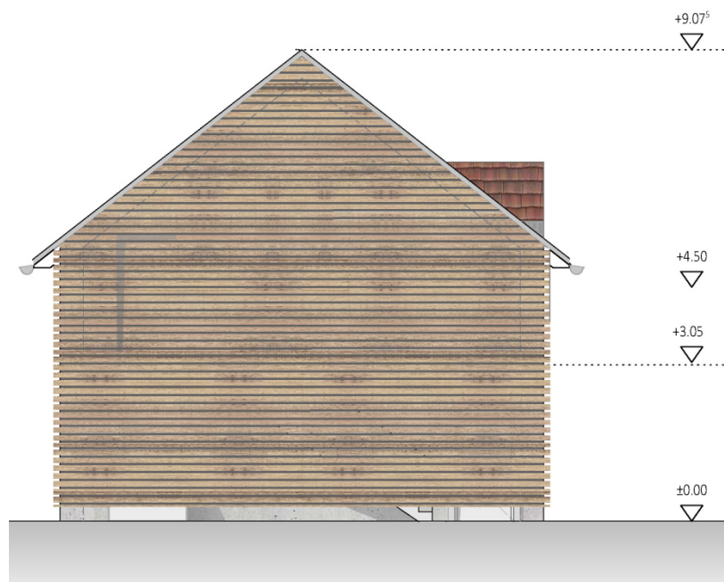
Westansicht
