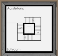
3.OG | +15.00
